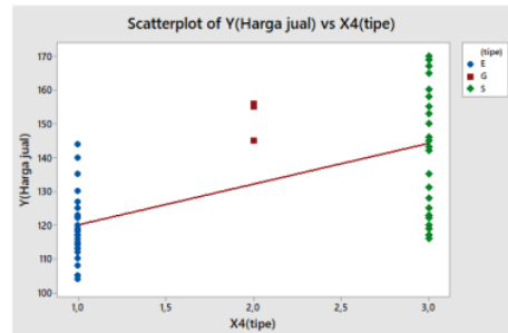
Gambar 7 Grafik persamaan regresi linear harga jual terhadap tipe mobil
