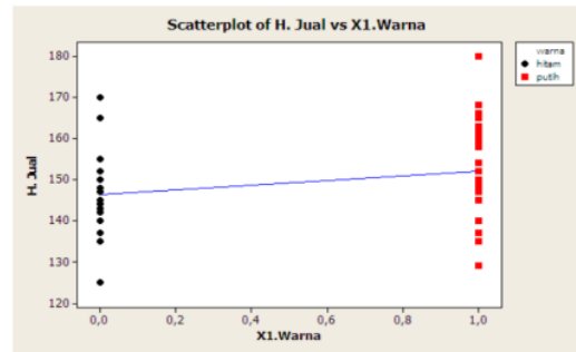
Gambar 3 Scatterplot Harga Jual Mobil Yaris terhadap Warna Mobil
