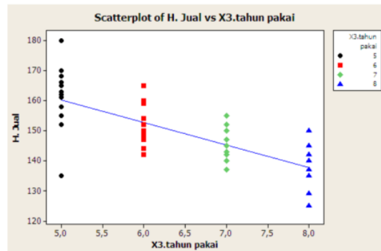
Gambar 10 Grafik persamaan regresi linear harga jual terhadap usia pakai (yaris)
