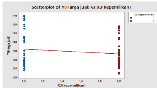
Gambar 5. Grafik persamaan Harga Jual terhadap kepemilikan (Yaris)
