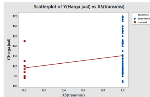
Gambar 8 Persamaan regrasi linear harga jual terhadap transmisi mobil
