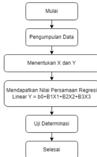
Gambar 1. Alur Desain Penelitian Regresi Linear
