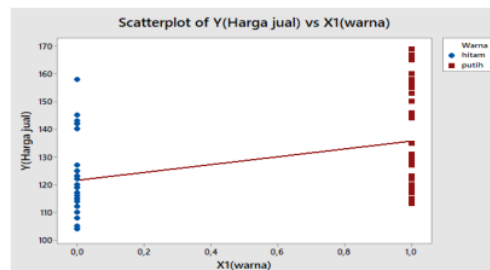
Gambar 4 Scatterplot Harga Jual Mobil Jazz terhadap Warna Mobil
