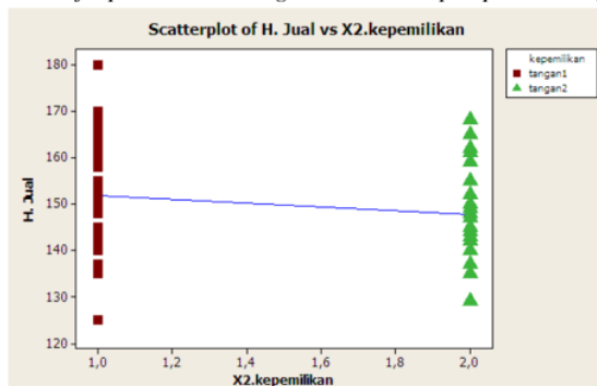
Gambar 6. Grafik persamaan Harga Jual terhadap kepemilikan (jazz)
